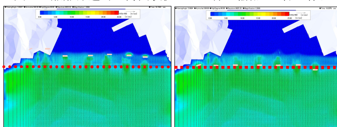
図-6 船舶浮遊時の流速分布 左：停止柵無し 右：有り
