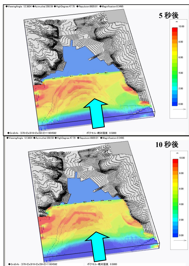
図-4 津波シミュレーション結果 押し波 海面状況 図-5 には船舶を湾内幅いっぱい複数隻配置した場合の、津波波力による流体-構造連成シミュレーション 2) の結果を示す。初期の津波段波よりも湾内に位置した船舶群は、押し波により更に湾内奥に浮遊するが、そ
