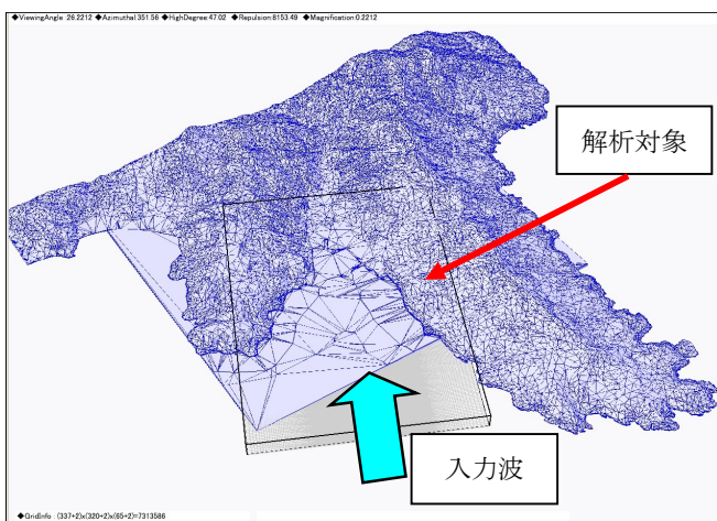
図-3 津波シミュレーションの解析領域
