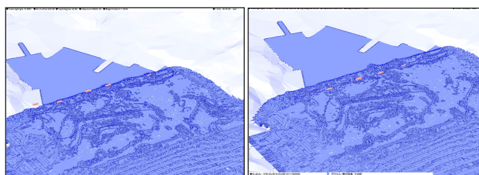
図-5 船舶浮遊時の海面状況 左：停止柵無し 右：有り
