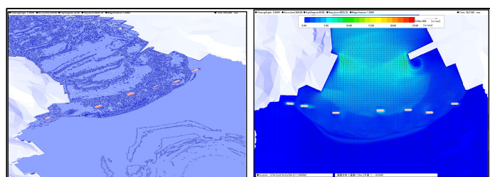
図-7 引波時の結果 左：海面状況 右：流速分布
